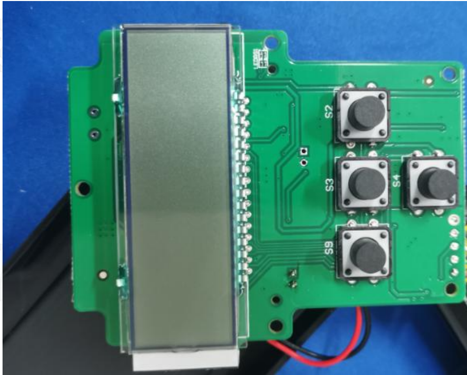
EUT Photo 5
